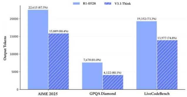
* 다양한 평가 지표의 점수가 유사한 상황에서 R1-0528과 V3.1-Think의 토큰 소비량 비교
